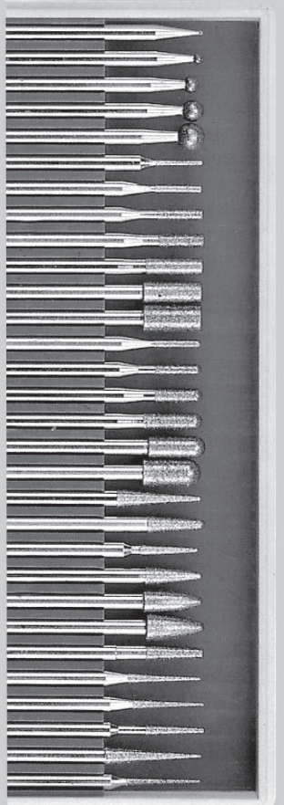
3mm Shaft
